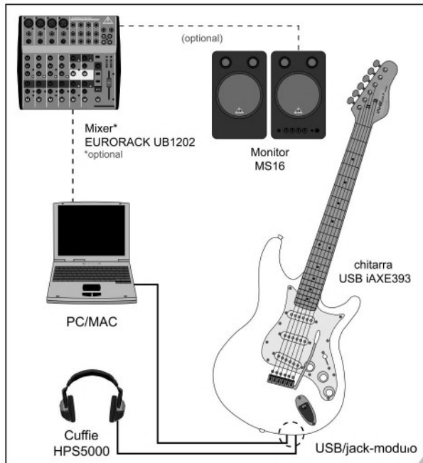
Fig. 4.1: Cablaggio della chitarra USB
