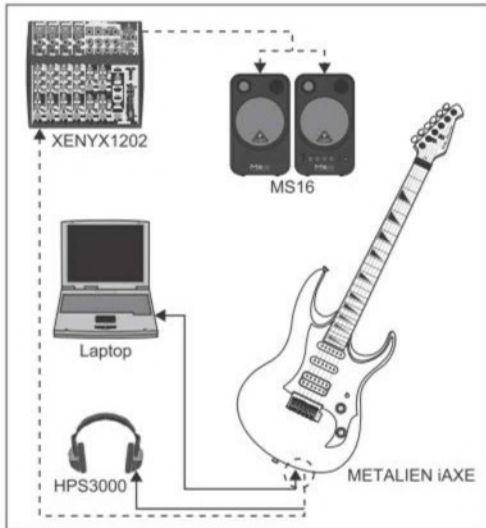
Abb. 4.1: Verkabelung der USB-Gitarre
