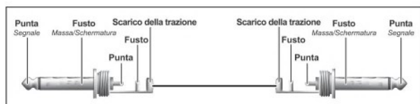
Fig. 5.1: presa mono jack 6,3-mm, asimmetrico
