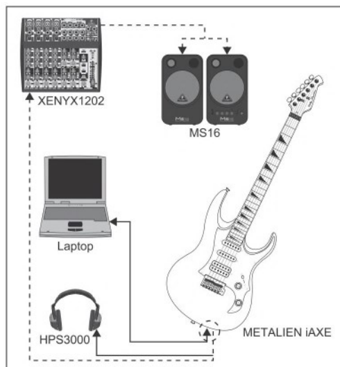
Fig. 4.1: Cablaggio della chitarra USB
